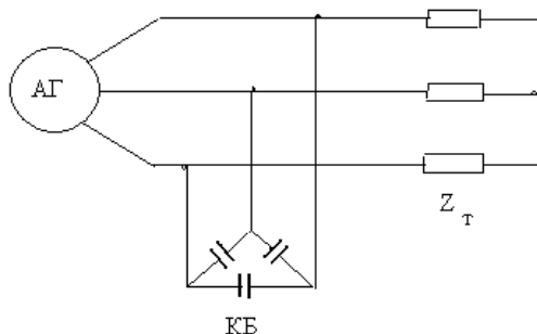
Фиг. 1. Принципна схема АГ
