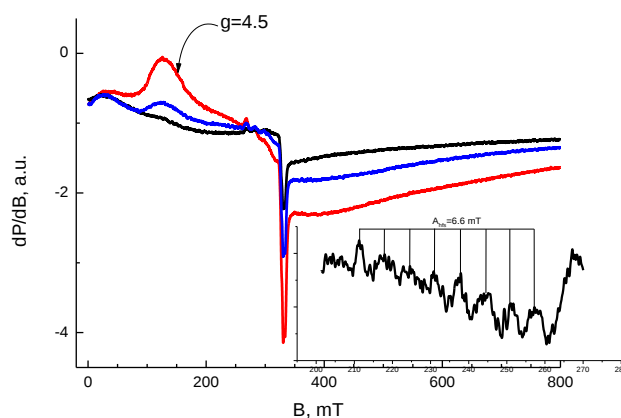
Фиг.2. ЕПР спектър на пигмент 0.3\text{CoO} \cdot 0.7\text{ZnO} \cdot \text{Al}_2\text{O}_3 след изпичане при 1100^\circ\text{C} и температури 100\text{K} (червена линия), 200\text{K} (синя линия) и 295\text{K} (черна линия)
