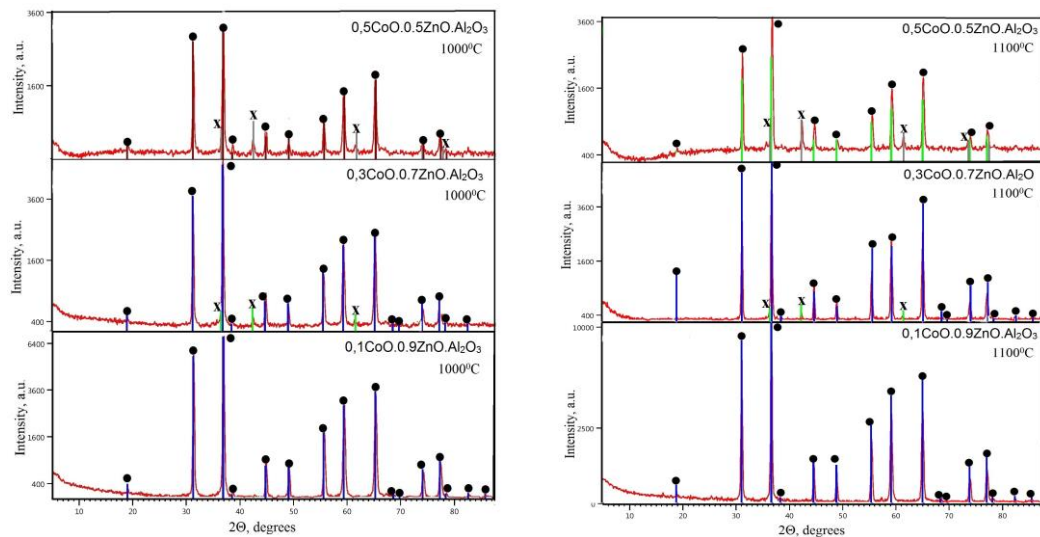
Фиг. 1. Рентгенограми на синтезирани шпинелни пигменти в системата x\text{CoO} \cdot (1-x)\text{ZnO} \cdot \text{Al}_2\text{O}_3 , където x=0,1; 0,3; 0,5 при 1000^\circ\text{C} и 1100^\circ\text{C} :
