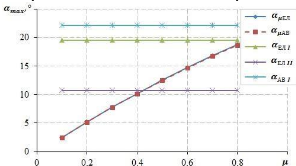
Фиг. 4. Ъгли на максимално преодоляван наклон в зависимост от коефициента на сцепление (4 човека + 40 kg)
