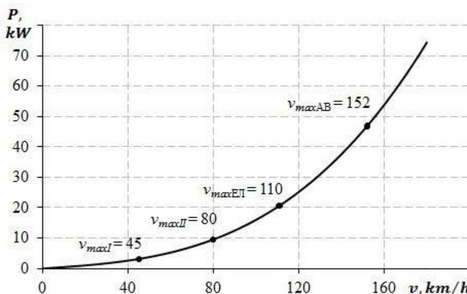
Фиг. 7. Максимална скорост на автомобила и на конвертирания електромобил
