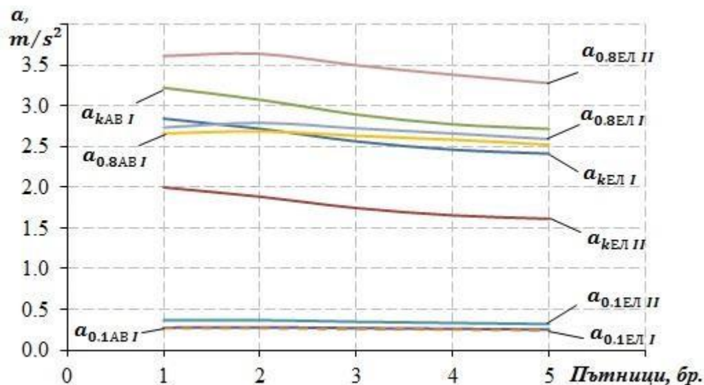
Фиг. 5. Максимални ускорения на автомобила (AB) и на електромобила (ЕЛ) Ускоренията се определят по следната формула:
