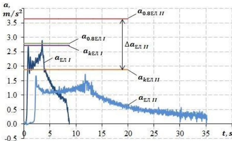
Фиг. 6. Ускорения, получени при пътни експерименти, сравнени с изчислените максимални стойности На фиг. 6 са представени ускоренията на електромобила на първа a_{\text{ЕЛ I}} и втора a_{\text{ЕЛ II}} предавка, получени при пътни експерименти. Те са сравнени с изчислените максимални
