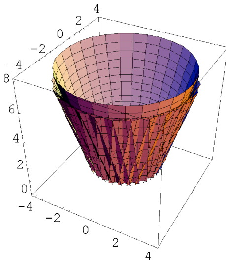
Фиг. 7 Параболоида и допирателните равнини при u = 1.5
