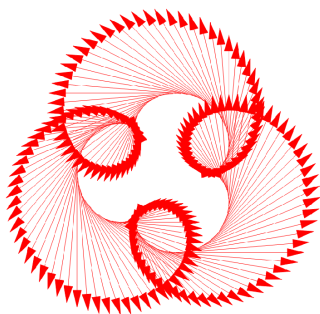
Фиг.2 Допирателно векторно поле към епициклоида
