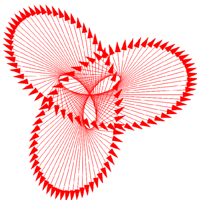
Фиг. 5 Допирателно векторно поле към трилистната роза
