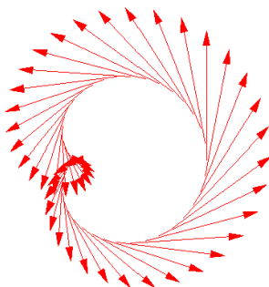
Фиг. 4 Допирателно векторно поле към кардиоида
