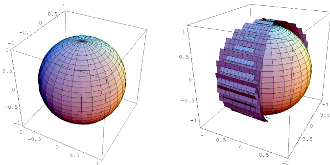
Фиг. 6 Единичната сфера и допирателни равнини към нея
