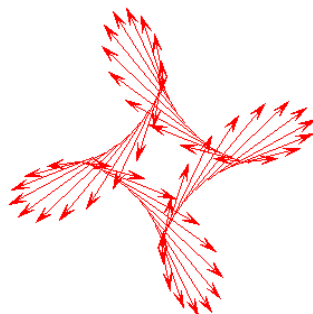
Фиг.3 Допирателно векторно поле към астроида
