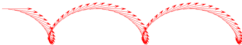
Фиг. 1 Допирателно векторно поле към циклоида
