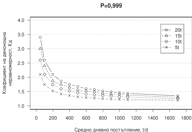
Фиг. 1. Коэффициенти на денонощна неравномерност в зависимост от средното дневно постъпление и средната товароносимост на превозните средства (5, 10, 15 и 20 t) при две нива на доверие - 0,95 и 0,999,
